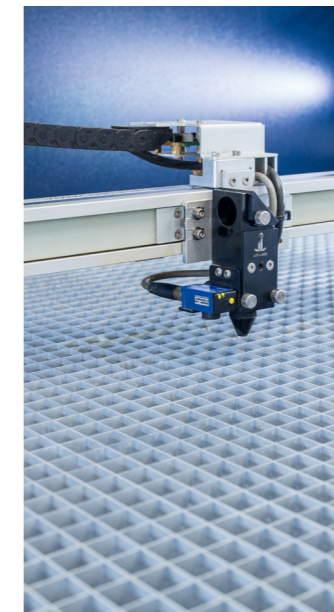
Gitterschneidertisch mit Vakuumpfunktion
