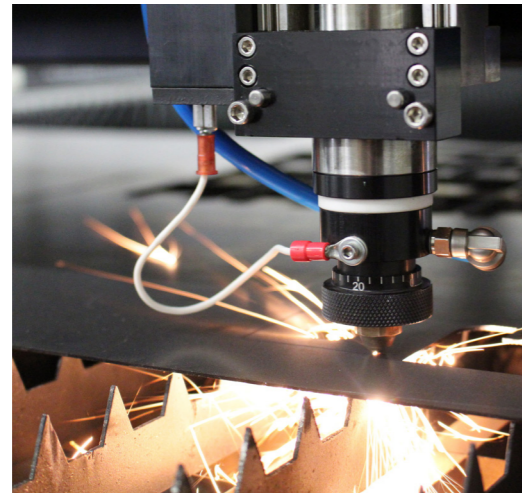
Metallschneideprozess
